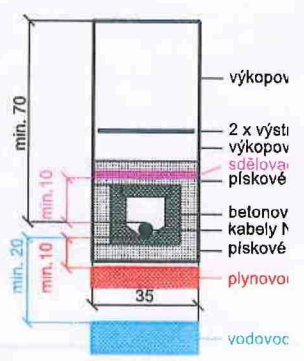
Křížení kabelu NN se sdělovým kabelem, plynovodem a vodovodem výkop 35 x 80 cm - volný teré
