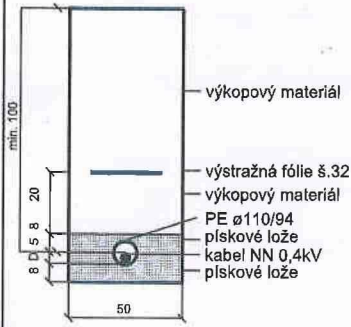
Uložení 1 kabelu NN ve volném terénu v chráničce "ŘEZ"
