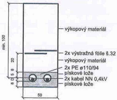
Uložení 1 kabelu NN ve volném terénu v chráničce "ŘEZ"
