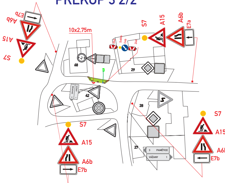
zábor vozovky:27,5m2
