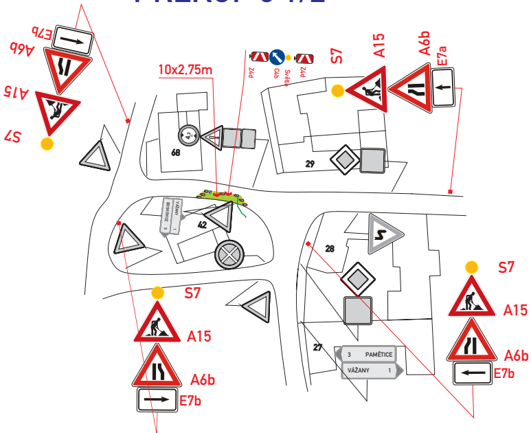
zábor vozovky:27,5m2
