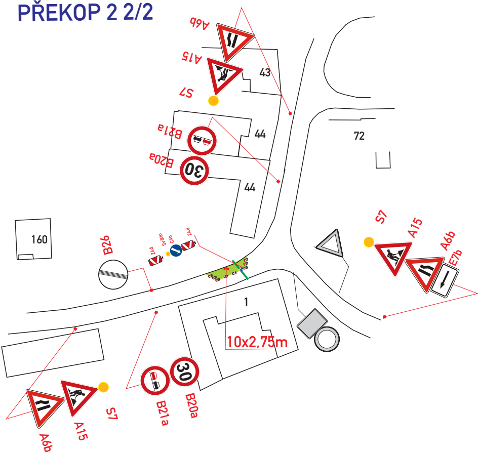
zábor vozovky:27,5m2
