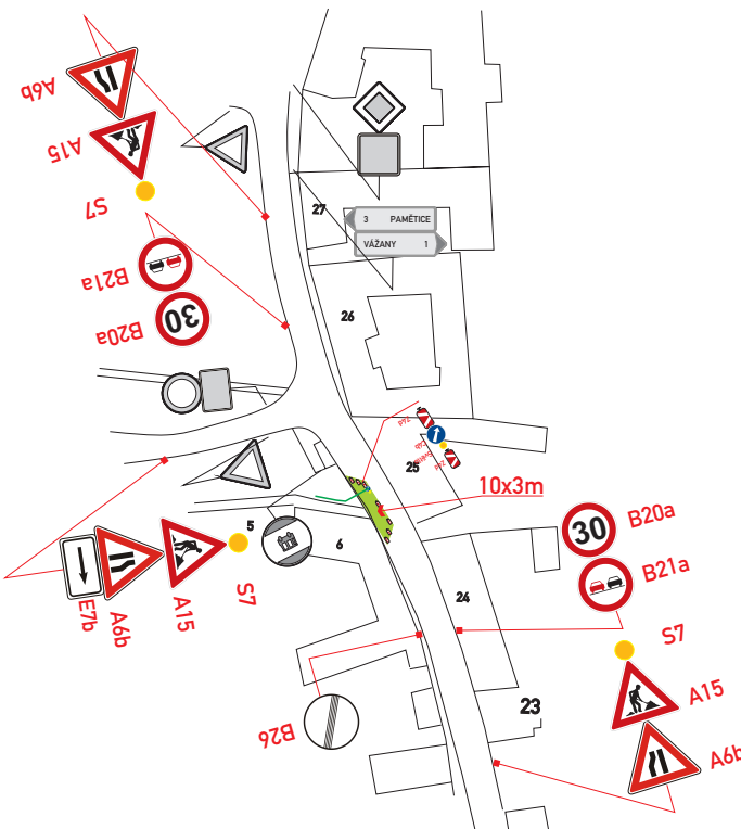
zábor vozovky:30m2
