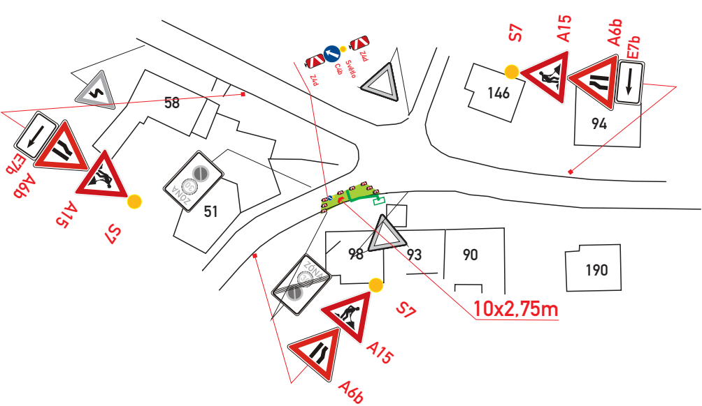
zábor vozovky:27,5m2
