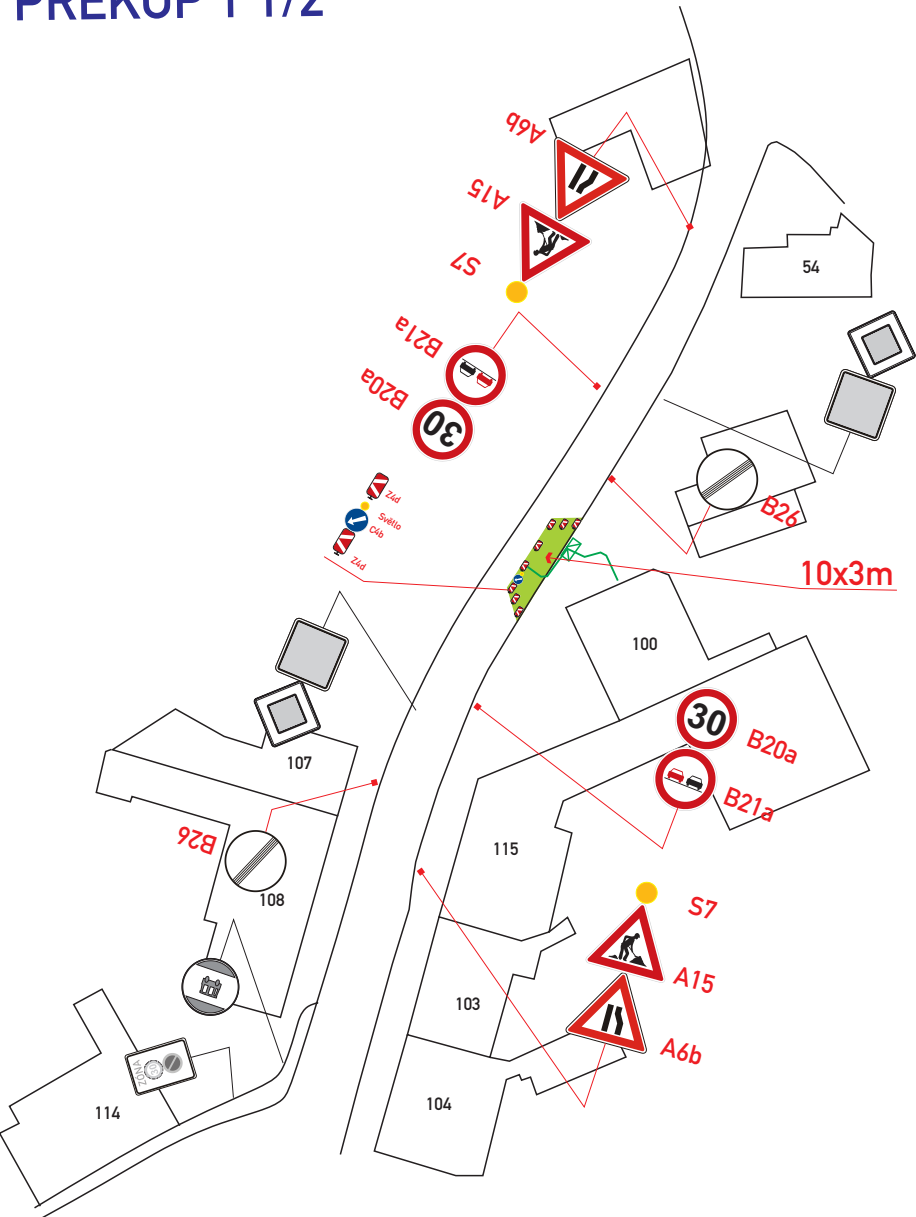
zábor vozovky:30m2
