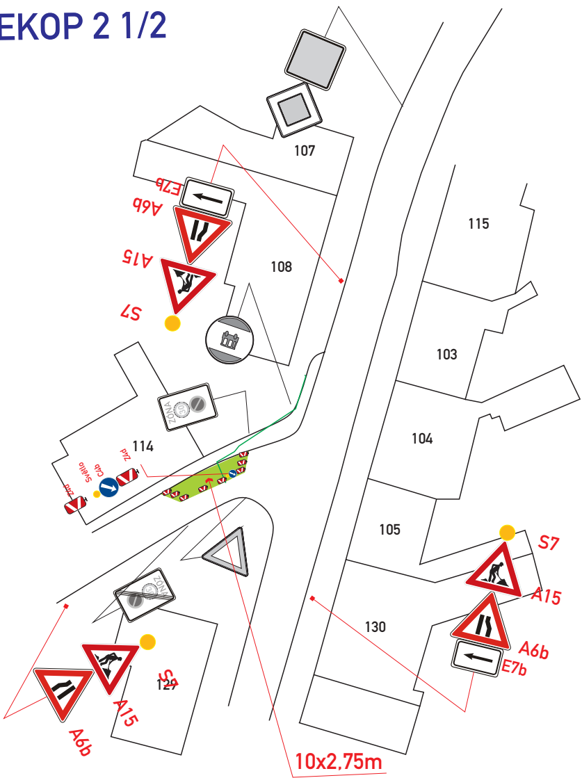
zábor vozovky:27,5m2
