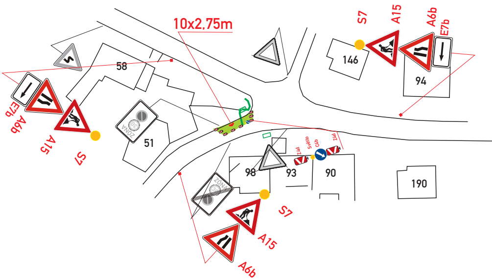
zábor vozovky:27,5m2
