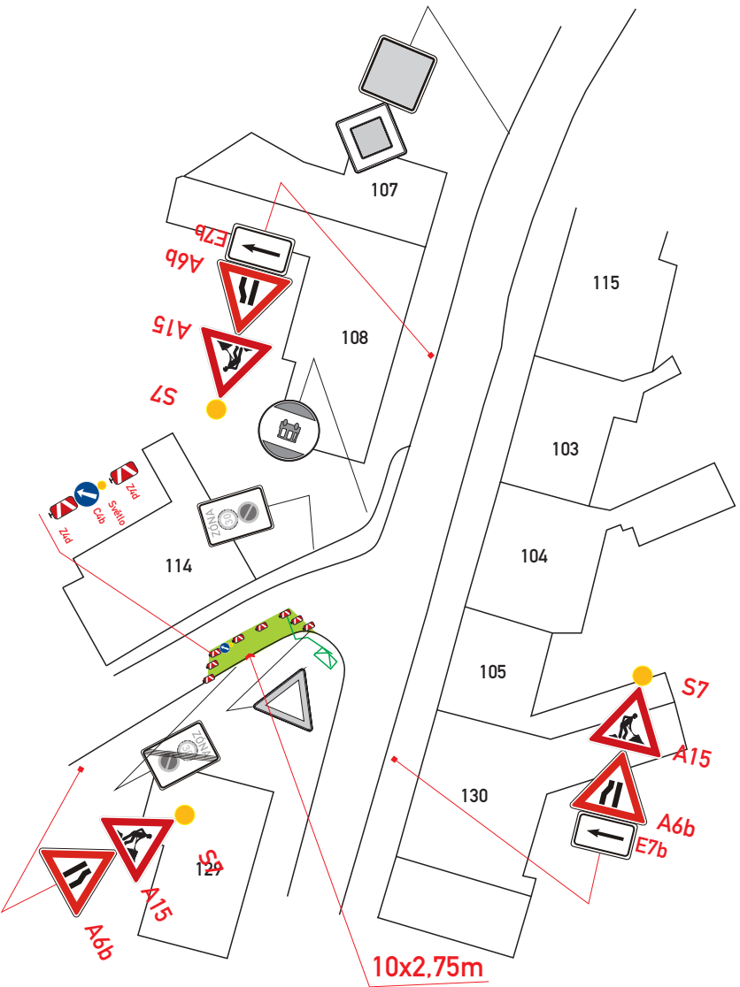
zábor vozovky:27,5m2
