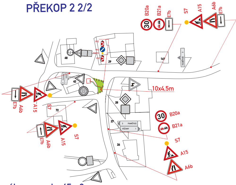
zábor vozovky:45m2
